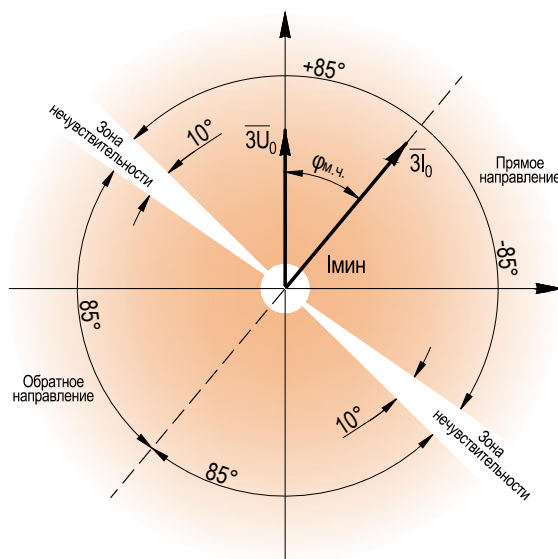
Рисунок 2.29 – Характеристика органа направления мощности нулевой последовательности
